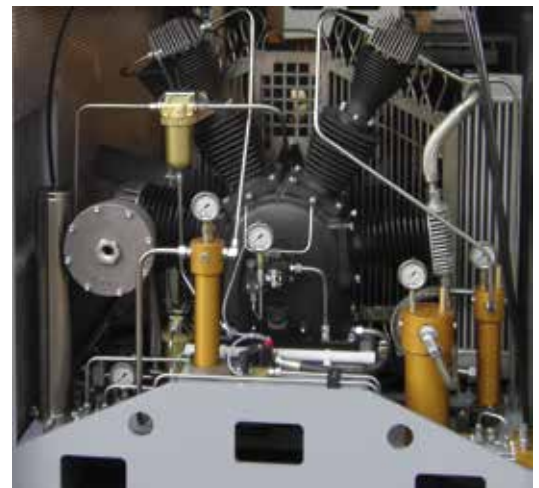
Schalldämmgehäuse LW 1300 E - Innenansicht
