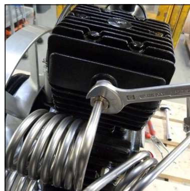
Abb. 6 - Rohrleitungsverschraubung
