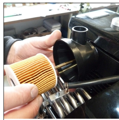
Abb. 5 - Ansaugfilter
