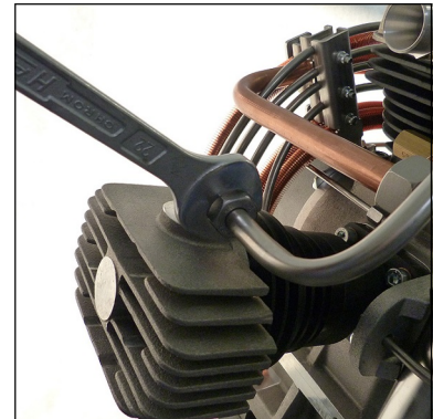
Abb. 1 - Rohrleitungsverraubungen lösen
