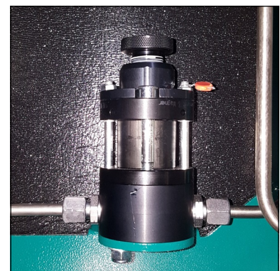
Sicherheitsventil 4. Stufe
