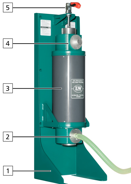
Abb. CO 2 Filter mit Standkonsole
